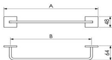
Toalheiro 30cm- A=348 B=300 07.QD02.CR 60cm- A=648 B=600 07.QD04.CR
