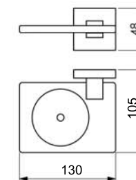
Saboneteira de Box 21.TS01.CR
