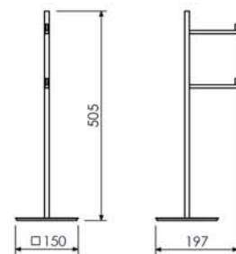
Coluna de Piso com Papeleira e Reserva 57.QD02.IP
