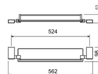
Porta Shampoo com Grade 29.OG01.CR
