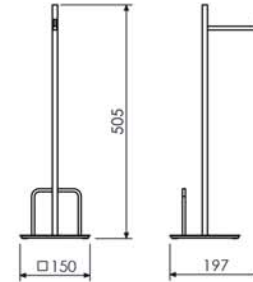
Coluna de Piso com Papeleira e Revisteiro 57.QD06.IP
