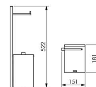
Coluna com Lixeira e Papeleira 57.QD05.IP
