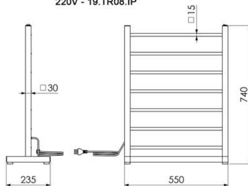
Toalheiro de Piso QUADA
