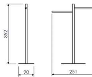
Toalheiro de Bancada Haste Dupla 17.QD01.CR
