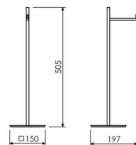
Coluna de Piso com Papeleira 57.QD01.IP
