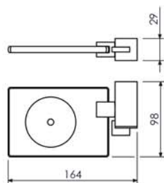
Saboneteira de Box 21.SQ01.CR
