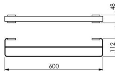
Toalheiro Duplo 60cm - 09.TS02.CR
