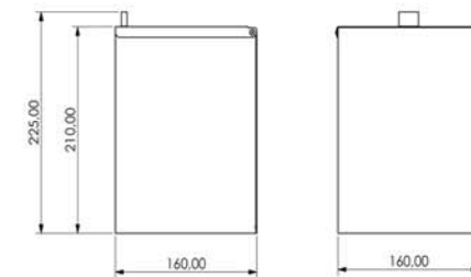
Lixeira Quadrada com Tampa 61.QD04.IP
