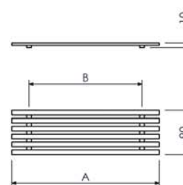
Saboneteira de Sobrepor 30cm - A=300 B=230 23.TW01.CR 35cm - A=350 B=280 23.TW02.CR 40cm - A=400 B=330 23.TW03.CR
