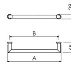
Toalheiro 30cm - A=329 B=300 07.PL02.CR 60cm - A=629 B=600 07.PL04.CR
