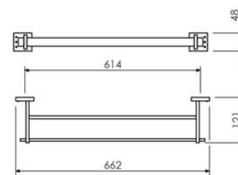
Toalheiro Duplo 60cm - 09.TB02.CR
