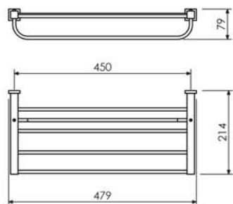
Toalheiro Rack com Alça 13.QD02.CR
