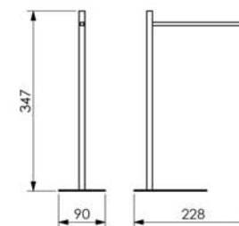
Toalheiro de Bancada Haste Simples 17.QD02.CR
