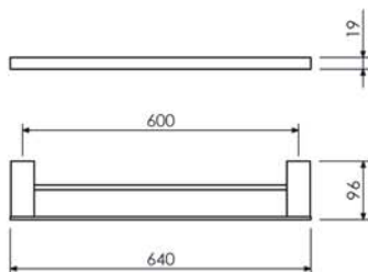
Toalheiro Duplo 09.UQ02.CR
