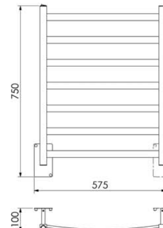
Sapphire Grande Fio Oculto 19.TS04.IP
