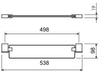
Porta Shampoo 29.UQ00.CR
