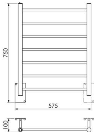
Ruby Grande Fio Oculto 19.TY04.IP
