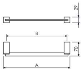
Toalheiro 30cm - A=329 B=300 07.SQ02.CR 60cm - A=629 B=600 07.SQ04.CR
