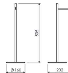
Coluna de Piso com Papeleira 57.RD01.IP
