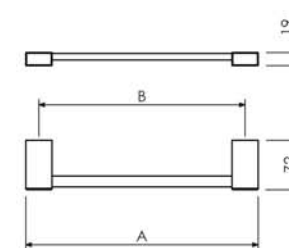
Toalheiro 20cm A=238 B=200 07.OG01.CR 30cm A=338 B=300 07.OG02.CR 45cm A=488 B=450 07.OG03.CR 60cm A=638 B=600 07.OG04.CR
