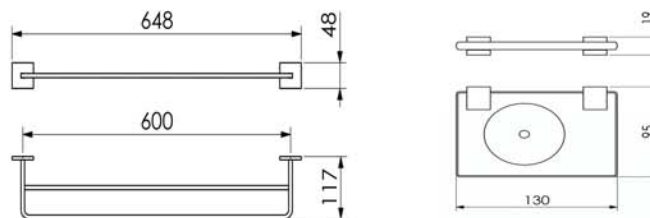
Toalheiro Duplo 09.QD02.CR
