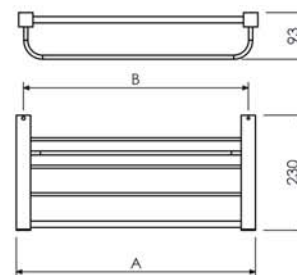
Toalheiro Rack com Alça 45cm - A=479 B=450 13.KP02.CR 60cm - A=629 B=600 13.KP06.CR
