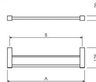
Toalheiro Duplo 45cm - A=479 B=450 09.KP01.CR 60cm - A=629 B=600 09.KP02.CR
