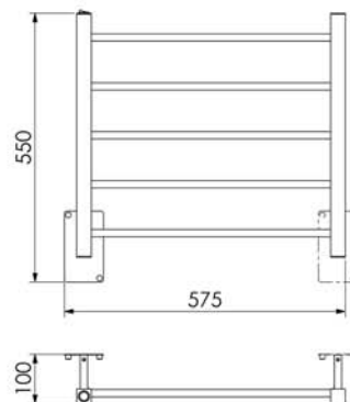
Quada Pequeno Fio Oculto 19.TQ02.IP
