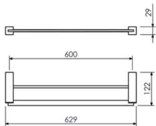
Toalheiro Duplo 09.SQ02.CR
