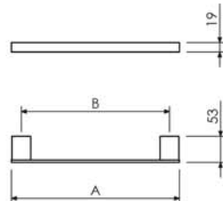
Toalheiro 30cm - A=340 B=300 07.UQ02.CR 60cm - A=640 B=600 07.UQ04.CR
