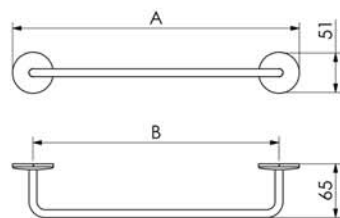
Toalheiro 30cm - A=351 B=300 07.RD02.CR 60cm - A=651 B=600 07.RD04.CR
