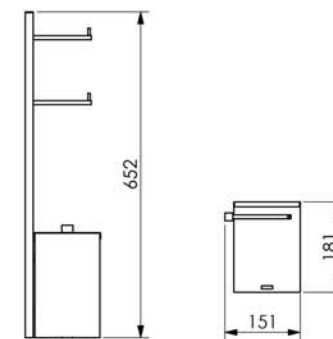
Coluna com Lixeira, Papeleira e Reserva 57.QD06.IP
