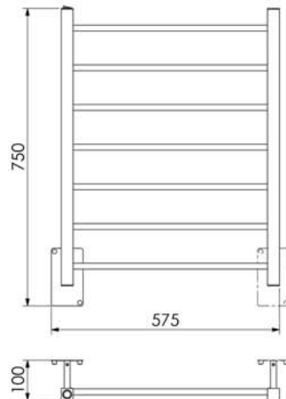
Quada Grande Fio Oculto 19.TQ04.IP
