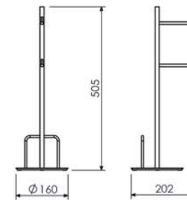
Coluna de Piso com Papeleira, Reserva e Revisteiro 57.RD04.IP
